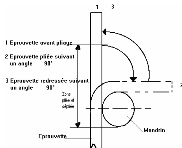
Figure 1 : Schéma descriptif de l'essai d'aptitude au redressage après pliage.
